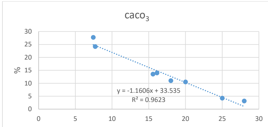
الشكل (5): العلاقة بين تركيز الفوسفور المتاح في التربة ومحتواها من كربونات الكالسيوم.
