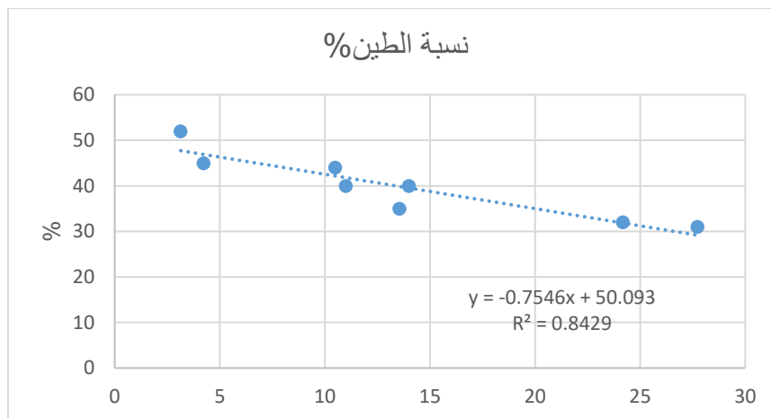
الشكل (6): العلاقة بين نسبة الطين في التربة ومحتواها من كربونات الكالسيوم
