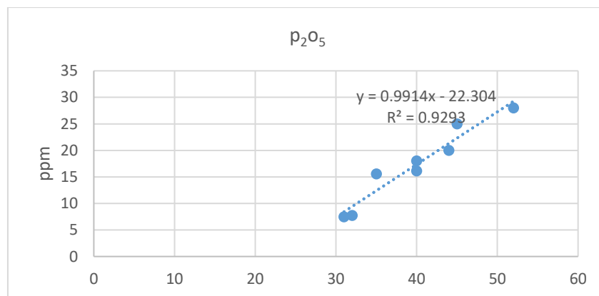
الشكل (7): العلاقة بين نسبة الطين في التربة ومحتواها من الفوسفور المتاح
