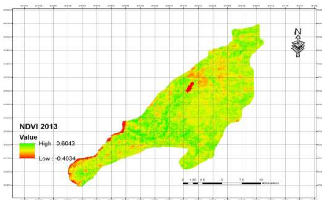
الشكل (2): قيم ال NDVI في منطقة الدراسة للعام 2013
