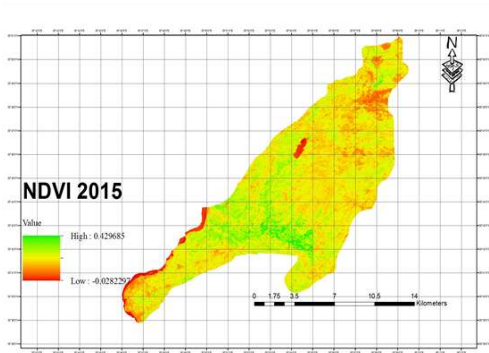
الشكل (3): قيم الـ NDVI في منطقة الدراسة للعام 2015
